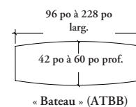
« Bateau » (ATBB)
