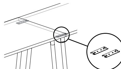
Avec plaques de liaison fixe
