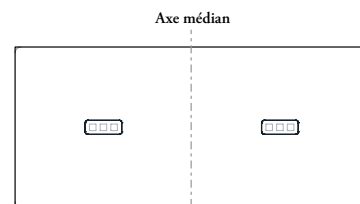
Découpe pour module affleurant – double (FD) et – triple (FT) (illustrée)
