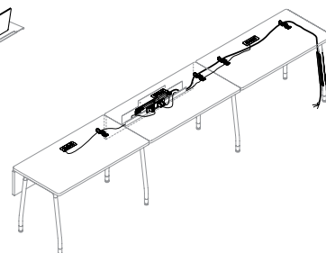
Câblage blindé
