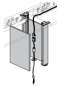
Base intermédiaire sans boîtier d'alimentation
