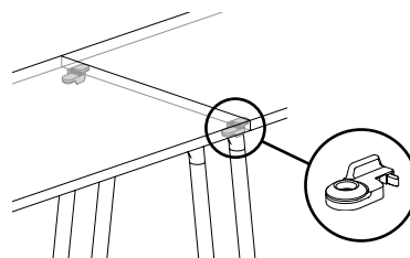
Avec dispositifs de liaison temporaire
