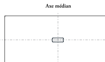
Découpe pour module affleurant – triple (FT)
