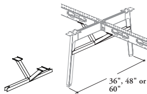
Double-Sided (D)
