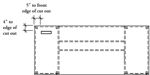
rectangular grommet
