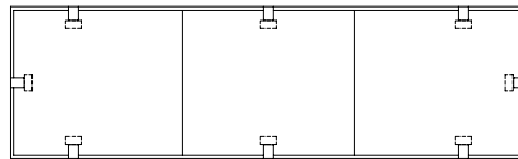
Edge USB Modules for 204" - 240" (8 modules)
